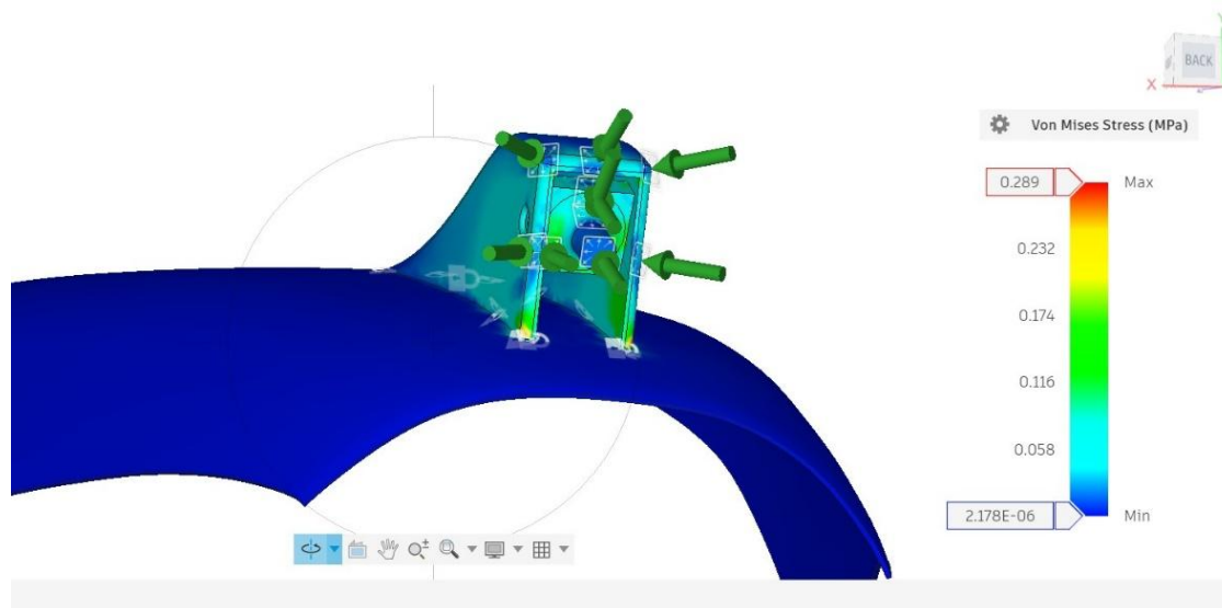
14 pav. Von Mises įtempia
