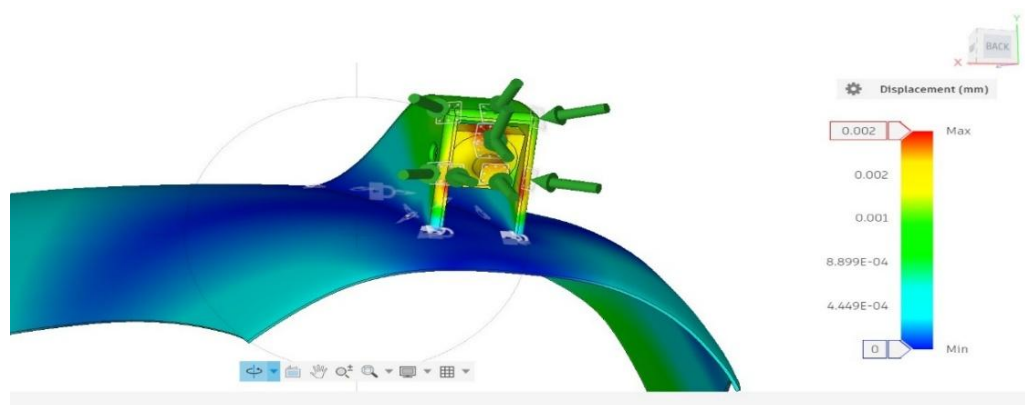
8 pav. Poslinkio vizualizacija
