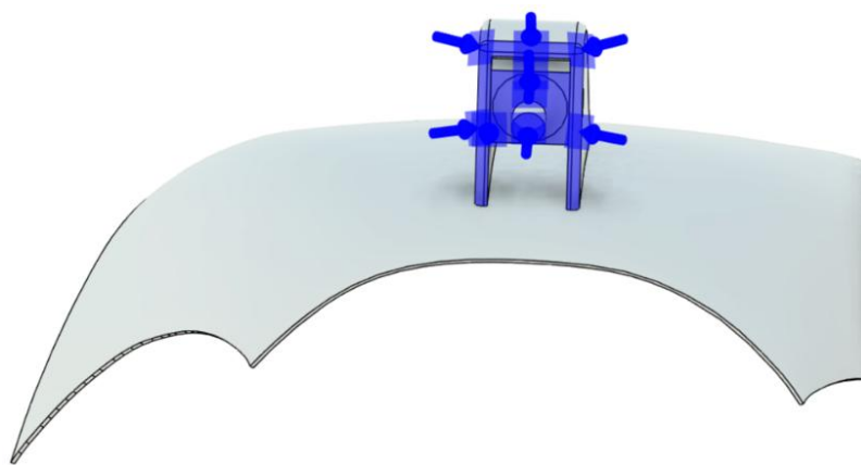
6 pav. Jėgos, veikiančios piloto kameros priekines briaunas Šaltinis: sudaryta autorių
