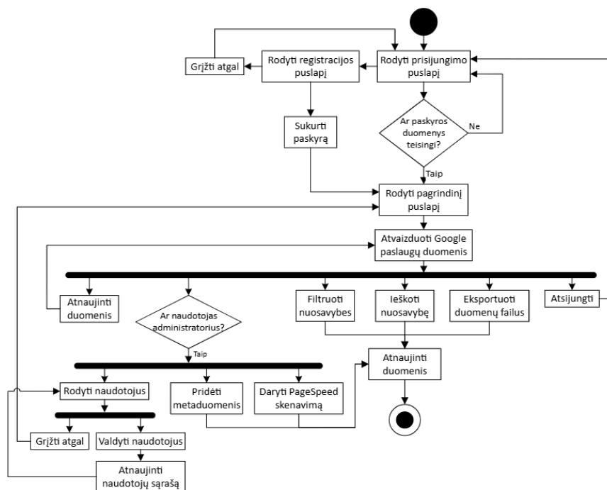
5 pav. Programos dinaminė vartotojo veiklos diagrama Šaltinis: sudaryta autorių
