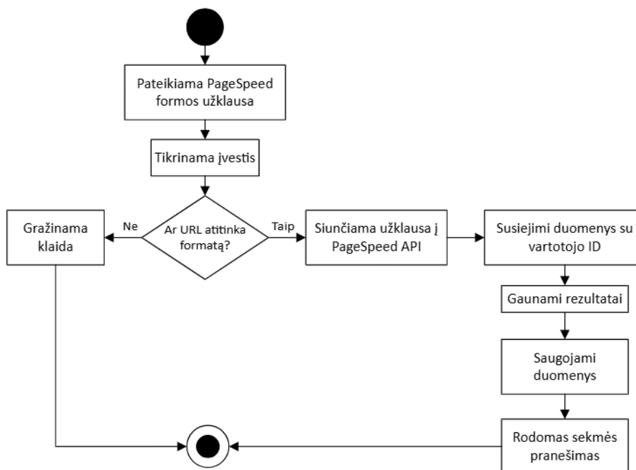
7 pav. PageSpeed nuskaitymo ir saugojimo algoritmo diagrama
