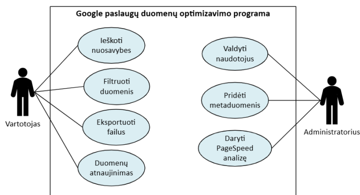
2 pav. Panaudojimo atvejų UML diagrama
