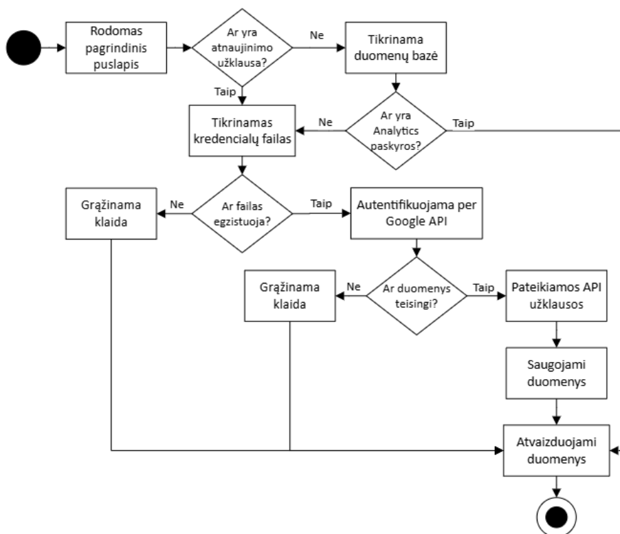
6 pav. Google Analytics duomenų sinchronizavimo algoritmo diagrama
