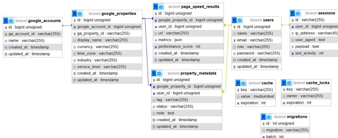
9 pav. Duomenų bazės lentelės ir jų santykiai per phpMyAdmin
