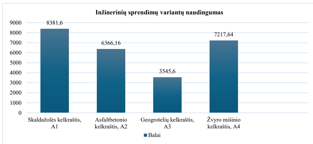
3 pav. Inžinerinių sprendinių variantų naudingumas, kai įvertintas teorinis kriterijų reikšmingumas
