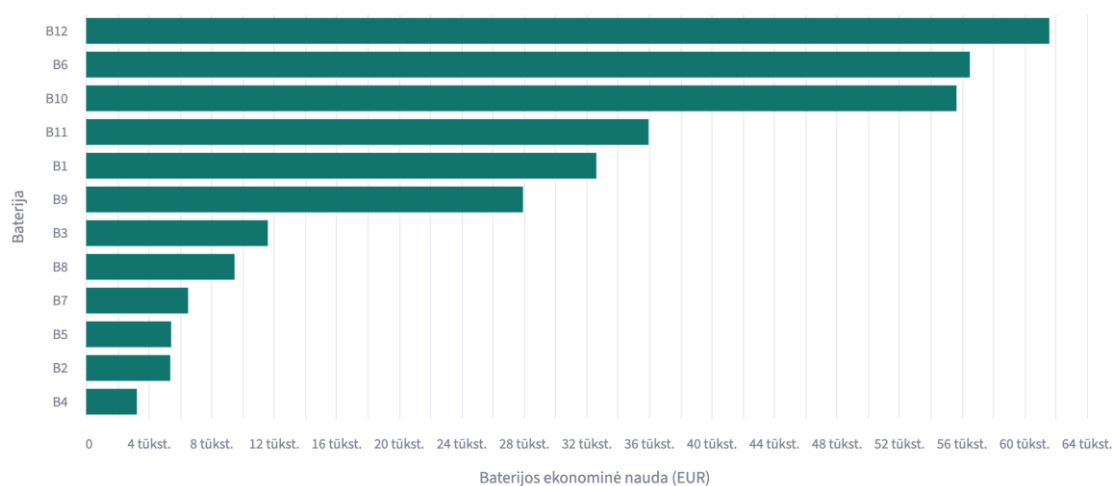
1 pav. Eksperimento metiniai rezultatai – baterijos ekonominė nauda
