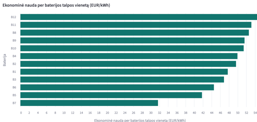
2 pav. Eksperimento metiniai rezultatai – baterijos ekonominė nauda per talpos vienetą Šaltinis: sudaryta autorių
