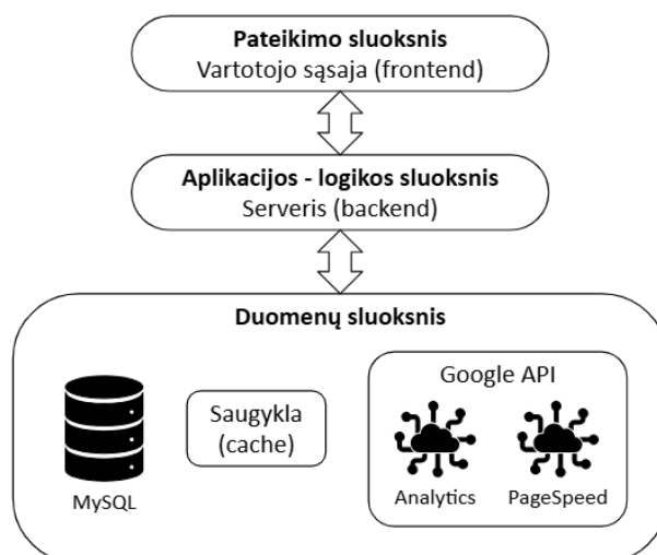
3 pav. Numatoma programos architektūros sprendimo diagrama
