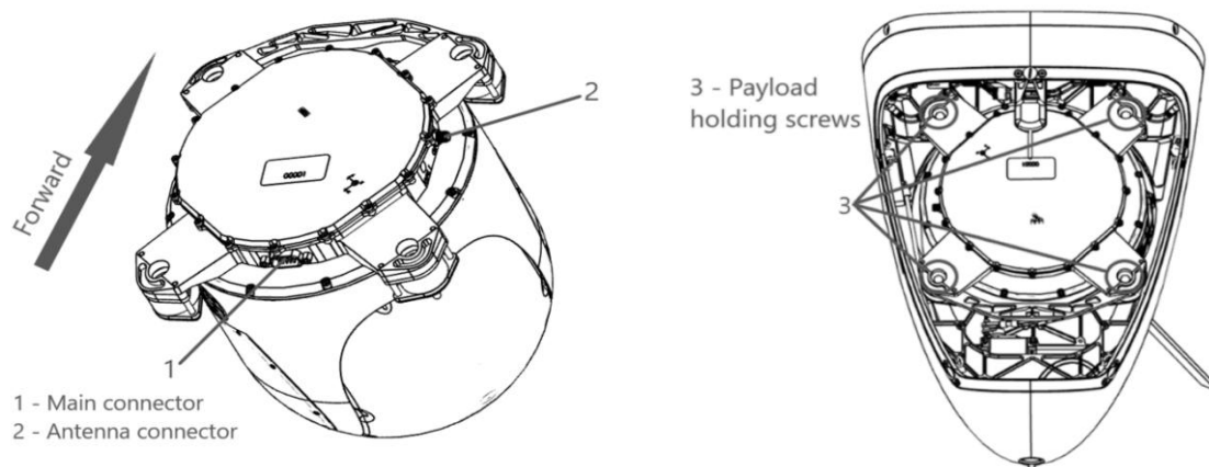
2 pav. Kameros tvirtinimo konstrukcija [1]
