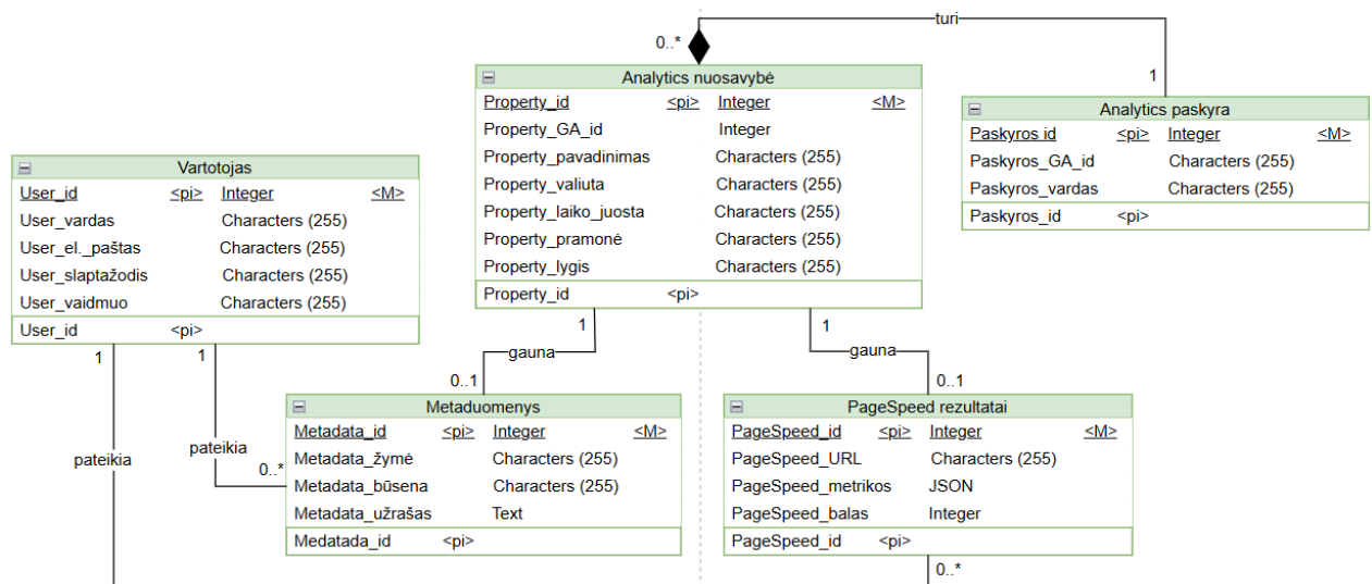
4 pav. Loginis duomenų modelis Šaltinis: sudaryta autorių
