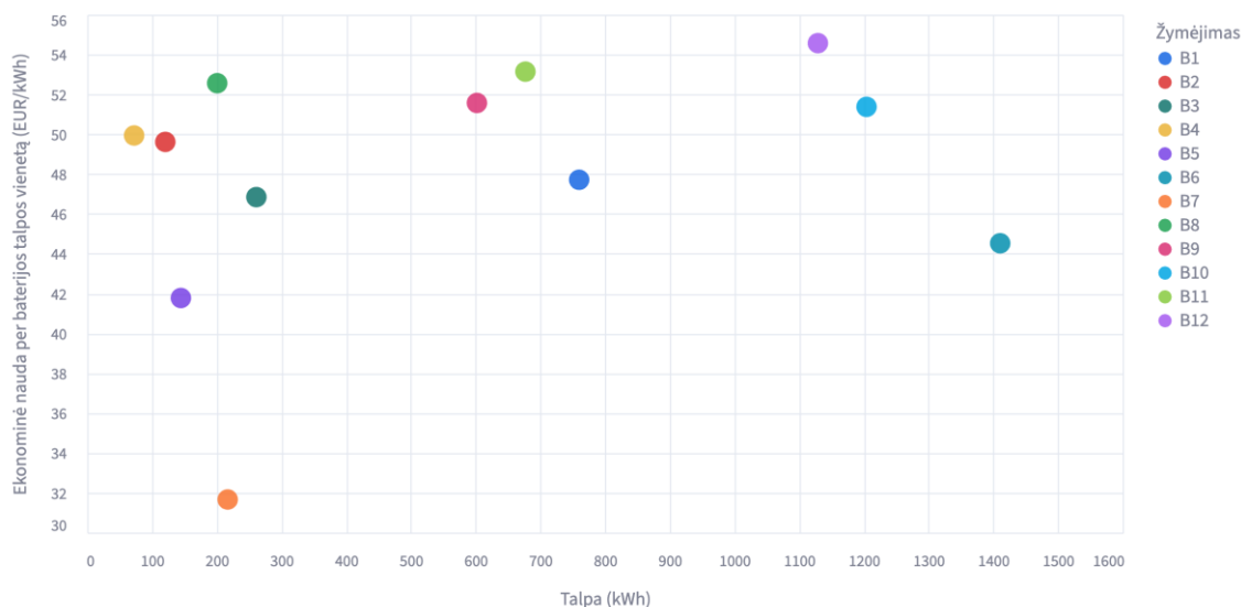
4 pav. Eksperimento metiniai rezultatai – baterijų ekonominio naudingumo išsidėstymo grafikas
