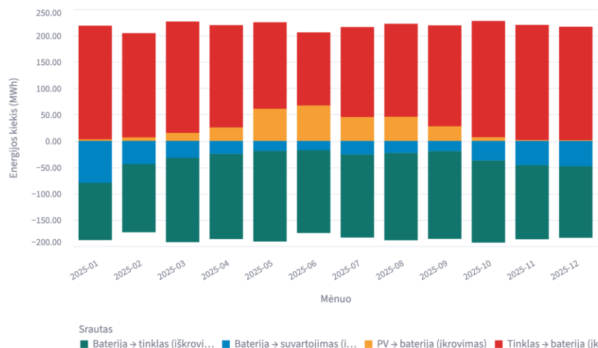
7 pav. Eksperimento metiniai rezultatai – suminiai baterijų energijos srautai
