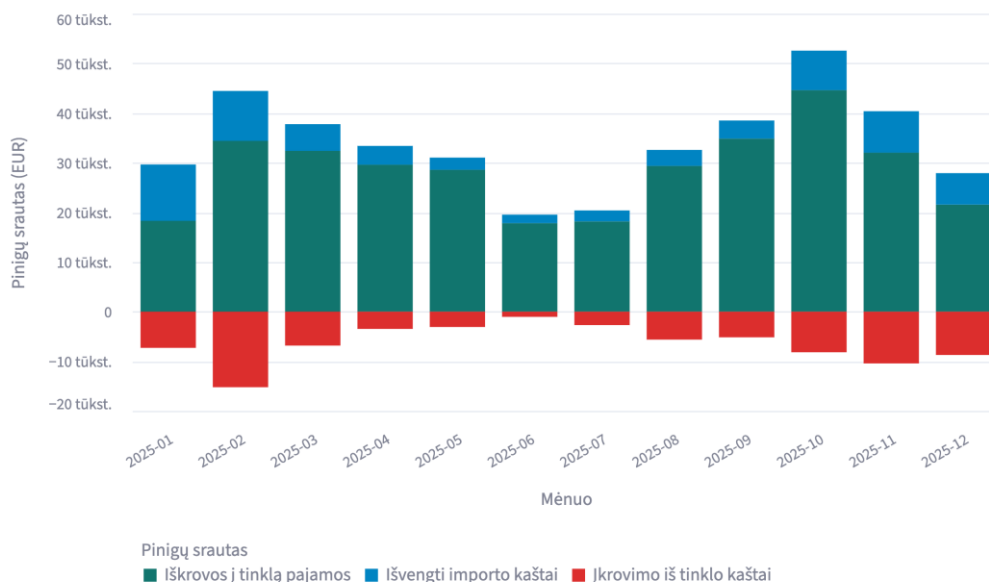
5 pav. Eksperimento metiniai rezultatai – suminiai pinigų srautai pagal mėnesį
