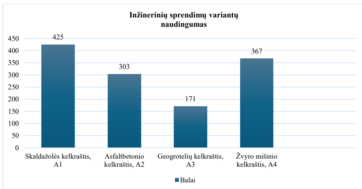
1 pav. Inžinerinių sprendimų variantų naudingumas, kai neįvertintas kriterijų reikšmingumas Šaltinis: sudaryta autorės
