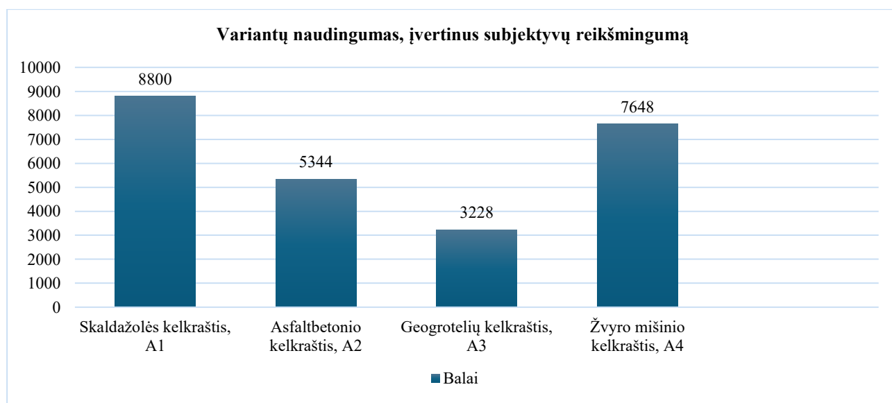
2 pav. Inžinerinių sprendimų variantų naudingumas, kai įvertintas subjektyvus kriterijų reikšmingumas Šaltinis: sudaryta autorės
