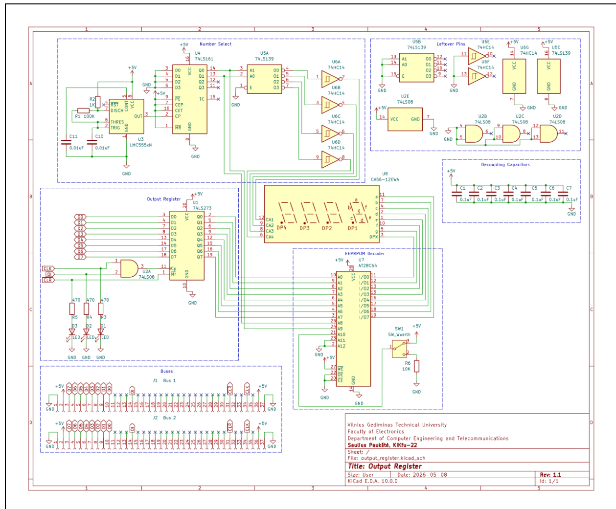
Fig. 14. Output register schematic
