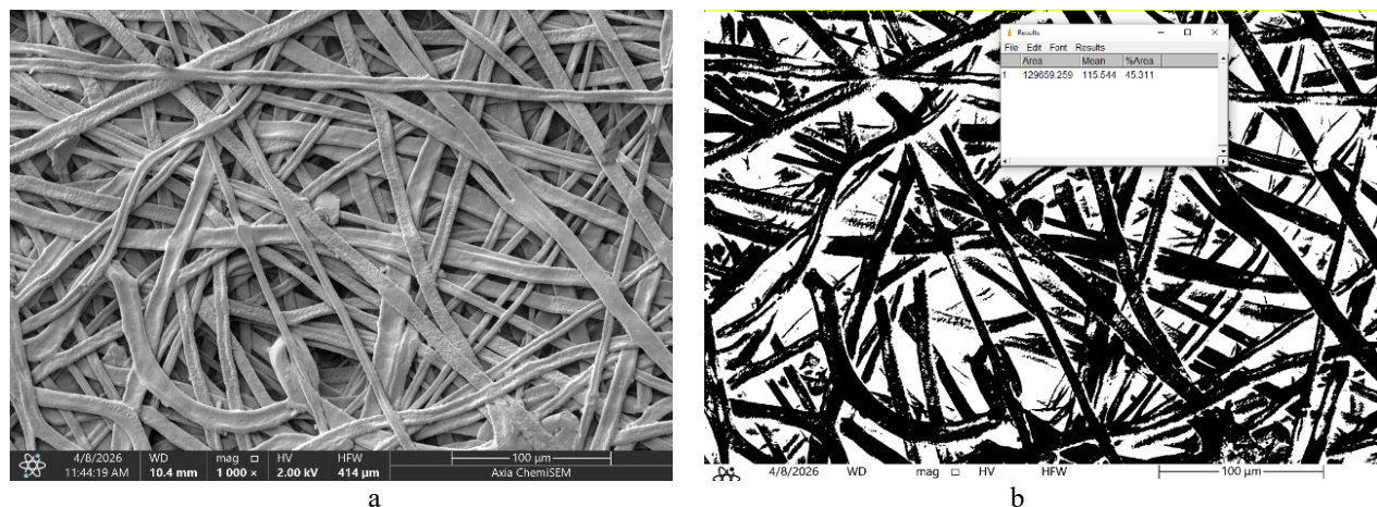
2 pav. PLGA nanopluosto morfologija: a – pradinė SEM nuotrauka; b – ImageJ programa apdorotas juodai baltas vaizdas, skirtas porėtumo analizei
