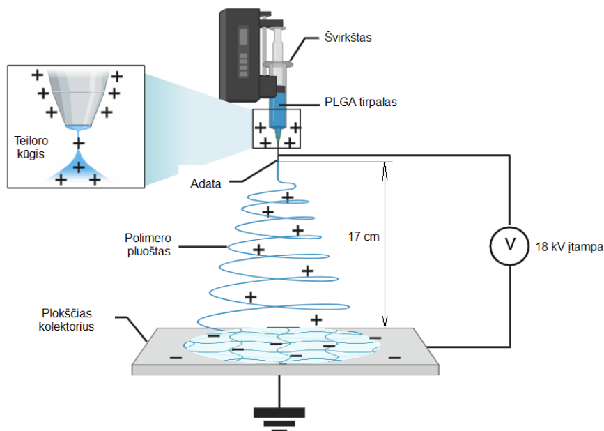
1 pav. PLGA nanopluošų gamybos elektroverpimo būdu schema
